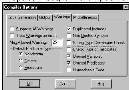
Рис.6. Установки опций компилятора
