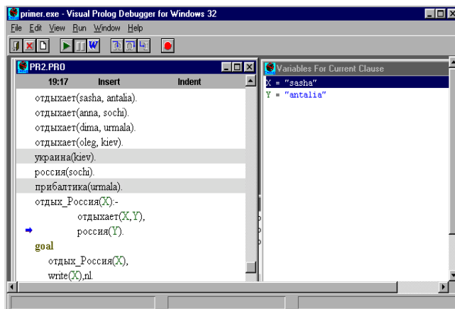
Рис.9. Окно отладчика
