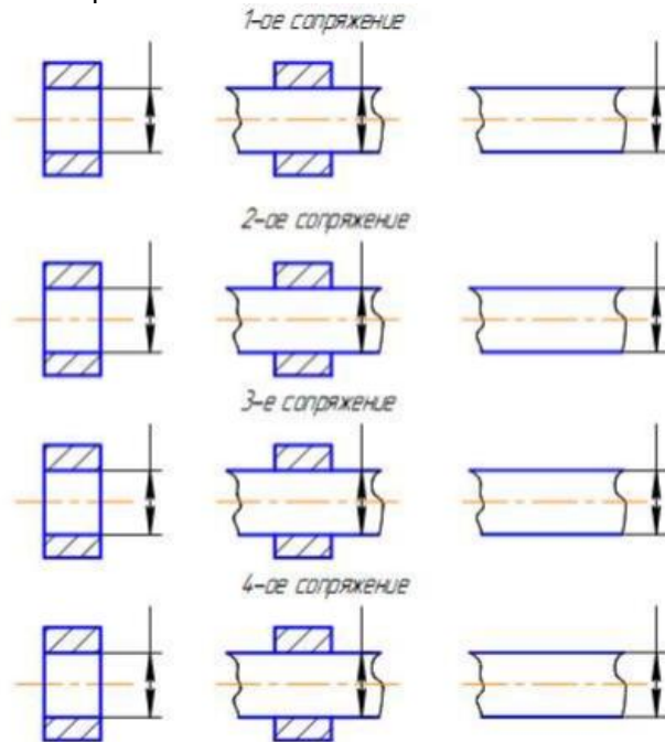
Рис. 2.6. Обозначение выбранных посадок на чертеже
