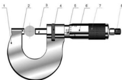
Рис. 1.1. Микрометр
