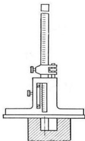
Рис. 1.2. Штангенглубиномер
