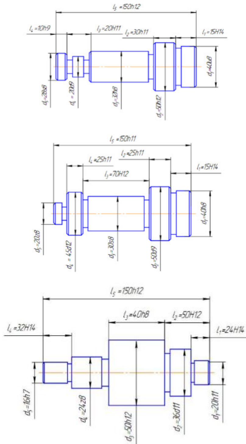
Рис. 1.5. Рабочий чертеж деталей
