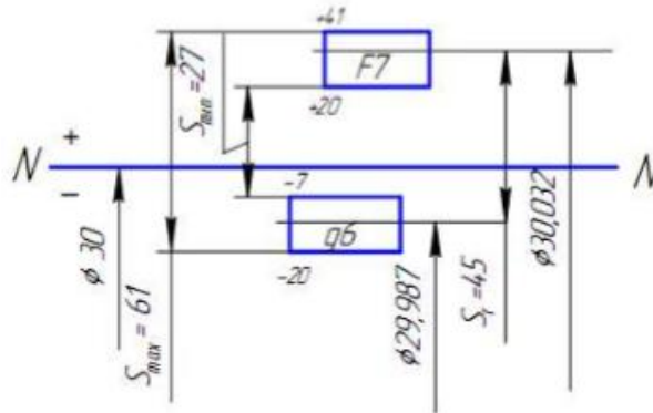
Рис. 2.4. Схема расположения полей допусков для заданного соединения
