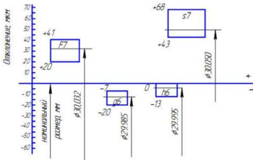
Рис. 2.5. Схема расположения полей допусков выбранных посадок
