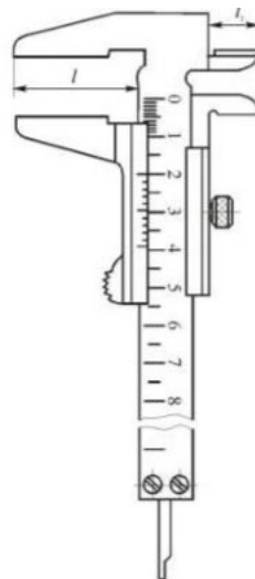
Рис. 1.3. Штангенциркуль
