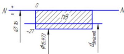
Рис. 1.4. Схема расположения поля допуска
