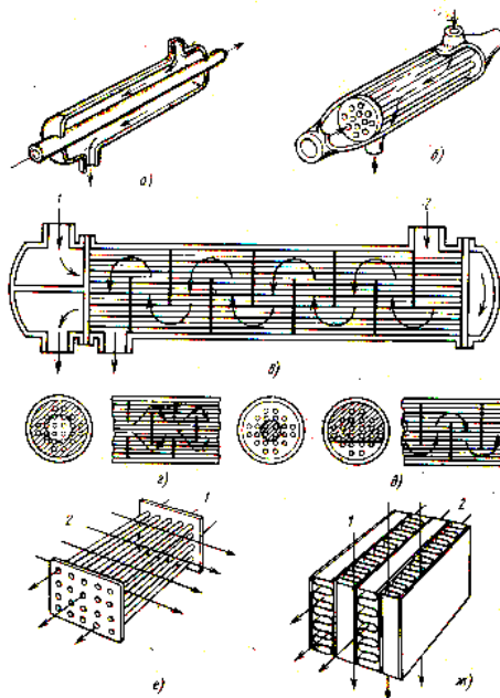
Рисунок 1 – Типичные конструктивные схемы рекуперативных теплообменных аппаратов а – «труба в трубе» противоток; б – кожухотрубный противоток; в, г, д – кожухотрубный многократный перекрестный ток; е- трубчатый перекрестный ток; ж – пластинчато-ребристый перекрестный ток; 1- горячий поток; 2 – холодный поток
