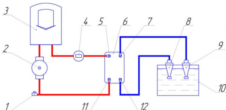
Рисунок 2 – Схема экспериментальной установки
